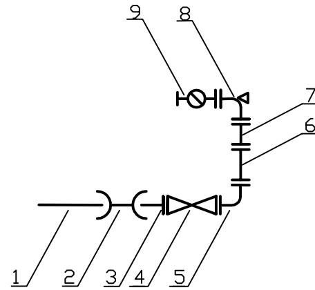
WĘZEŁ NR Hp28
